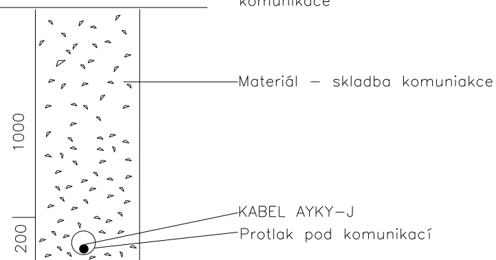
ŘEZ „ A ”
